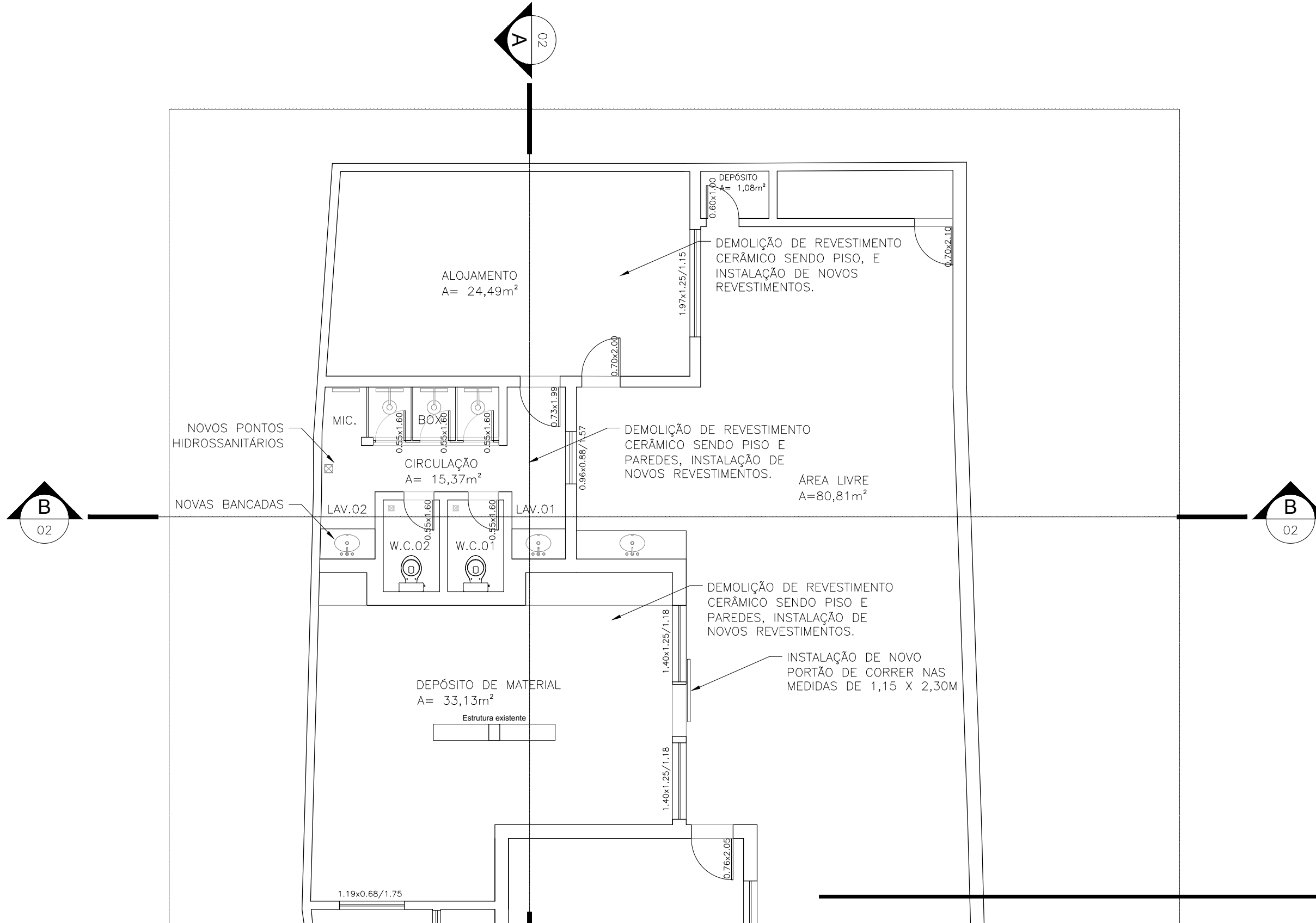
1 PLANTA BAIXA ESCALA 1:75
