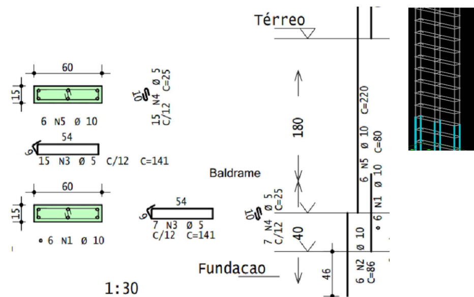
DETALHAMENTO PILAR P7 – CASA 02 SEM ESC.
