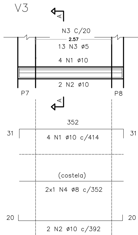
DETALHAMENTO DA VIGA BALDRAME E VIGA DE REFORÇO – CASA 02 SEM ESC.
