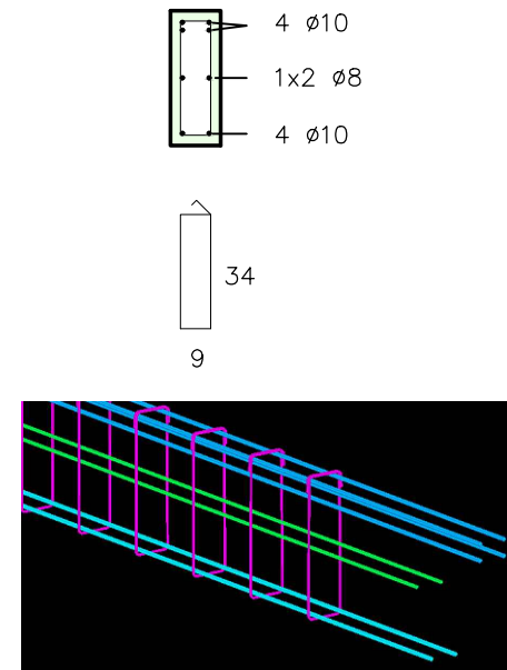
DETALHAMENTO DA VIGA BALDRAME E VIGA DE REFORÇO – CASA 02 SEM ESC.
