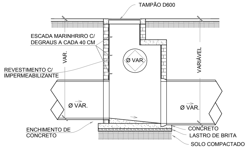
CORTE AA' SEM ESCALA
