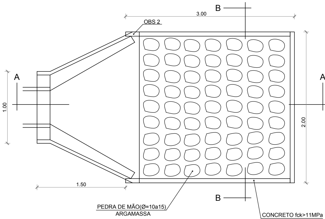
PLANTA BAIXA SEM ESCALA
