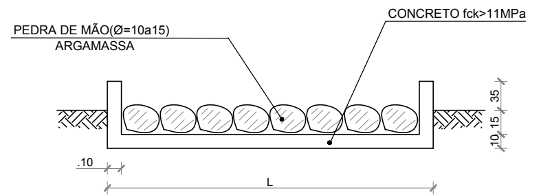
CORTE BB' SEM ESCALA
