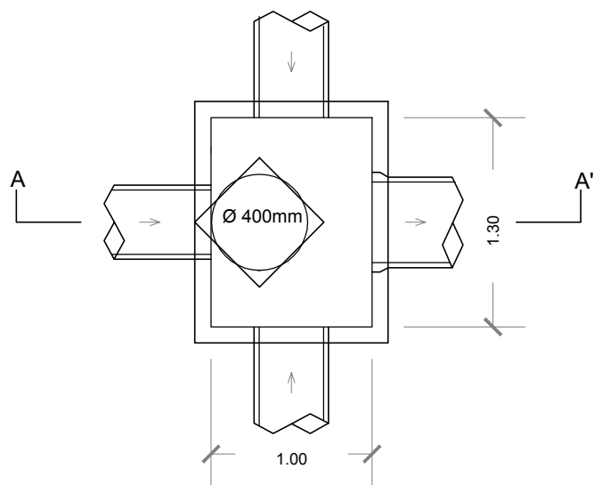
POÇO DE VISITA (PV) DE ÁGUA PLUVIAL TIPO1 - H= ACIMA DE 1,05 A 1,50M
