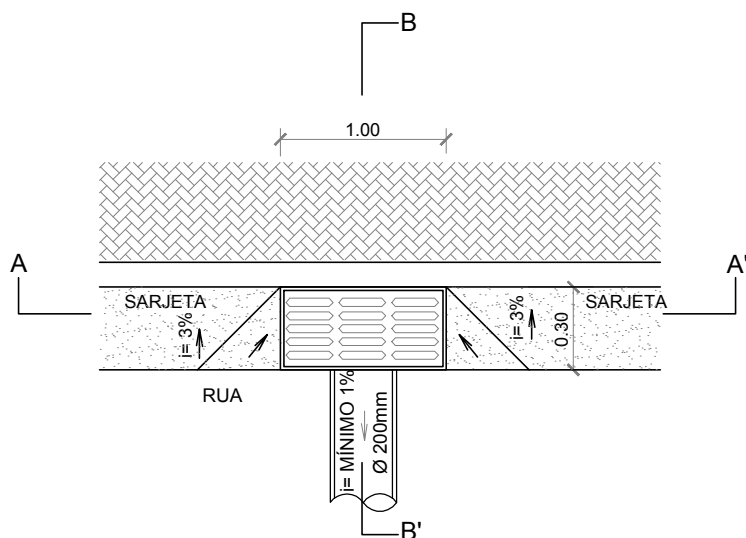
PLANTA BAIXA - BOCA DE LOBO SEM ESCALA
