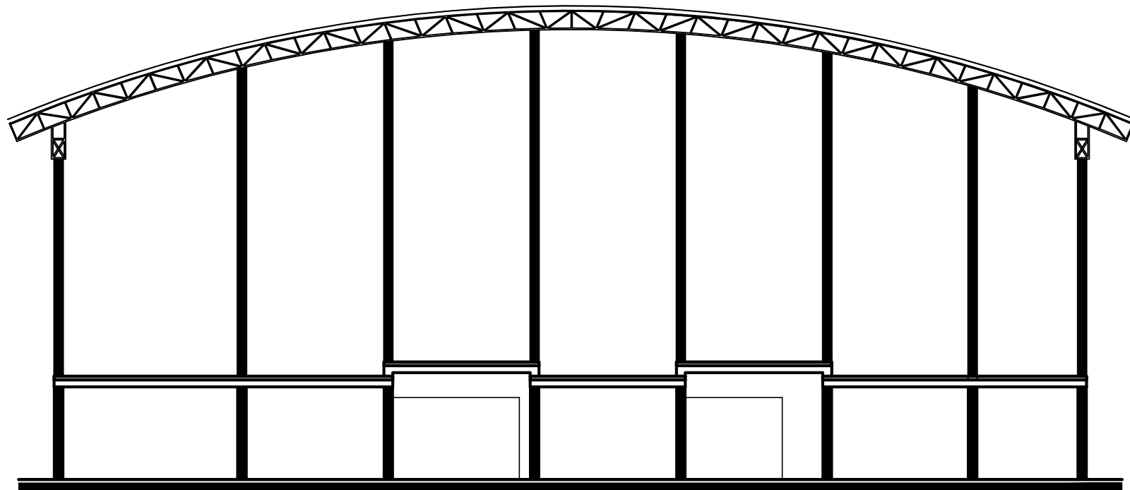
FACHADA FRONTAL esc 1:150
