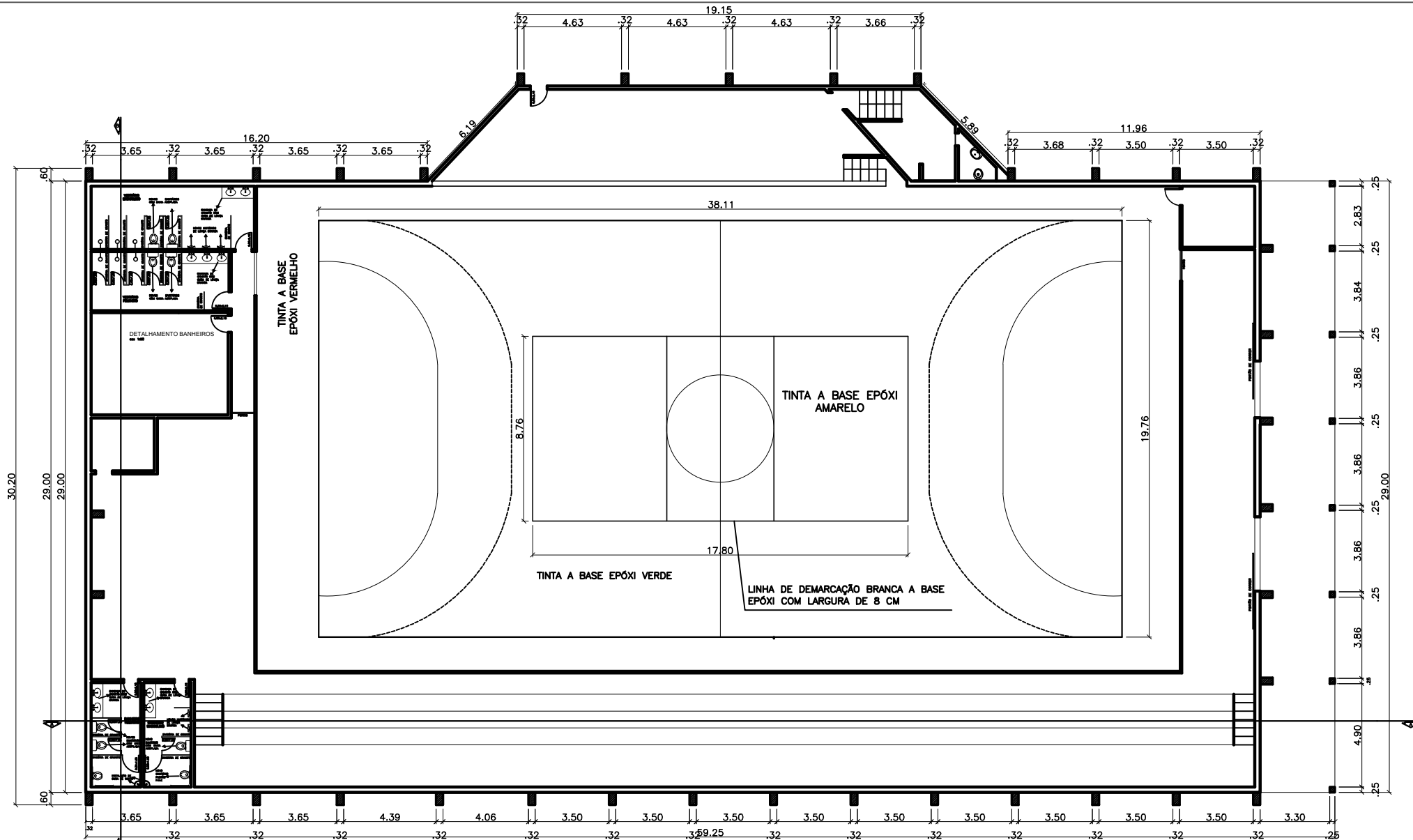
PLANTA DE REFORMA esc 1:250
