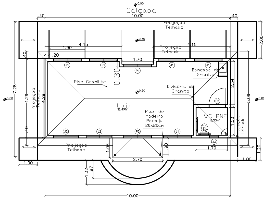
PLANTA BAIXA ESCALA 1 / 100
