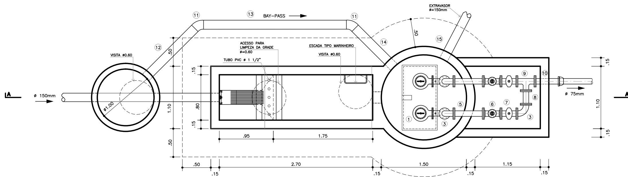
PLANTA BAIXA - ELEVATÓRIA/CX DE AREIA ESCALA: 1/25
