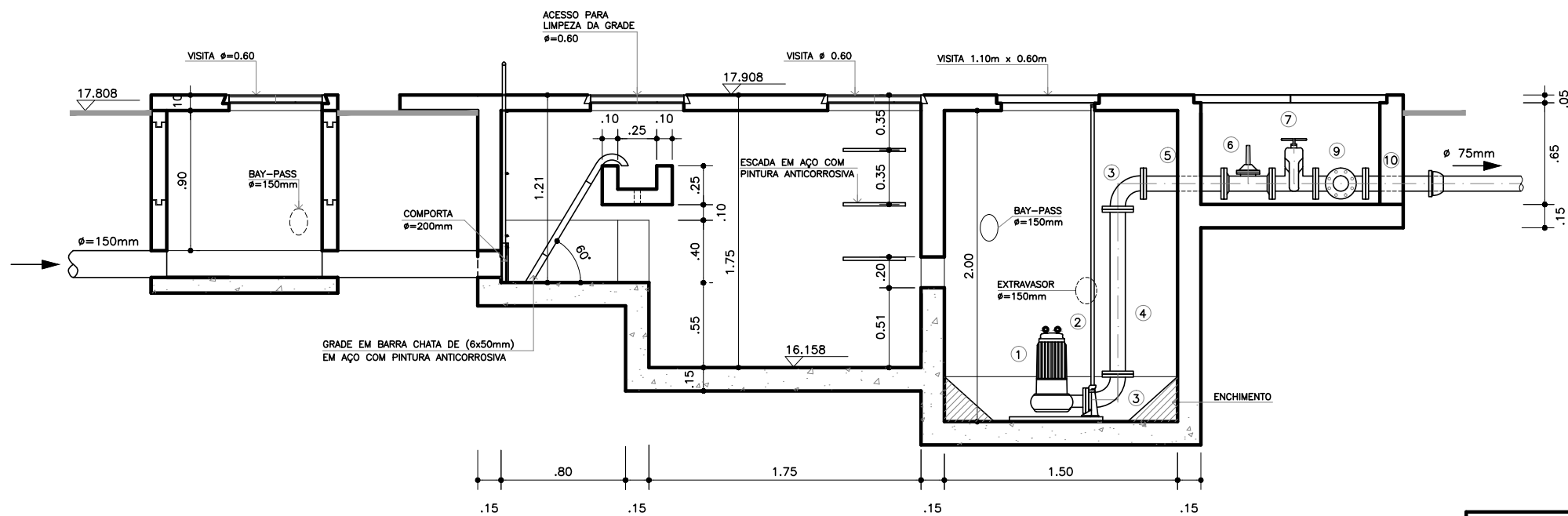
CORTE AA - ELEVATÓRIA/CX DE AREIA ESCALA: 1/25
